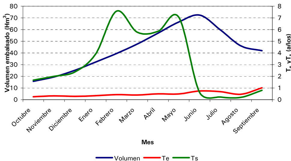
Figura 1: Volumen embalsado y tiempo de retención del agua
